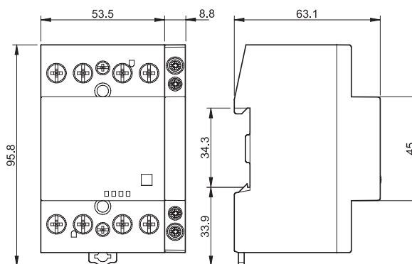
Tipo 22.44/22.64 + 022.63/022.65 Conexão a parafuso
