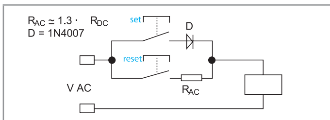
Circuito de comutação em AC
