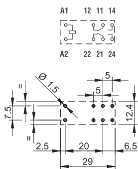
Vista do lado do cobre
